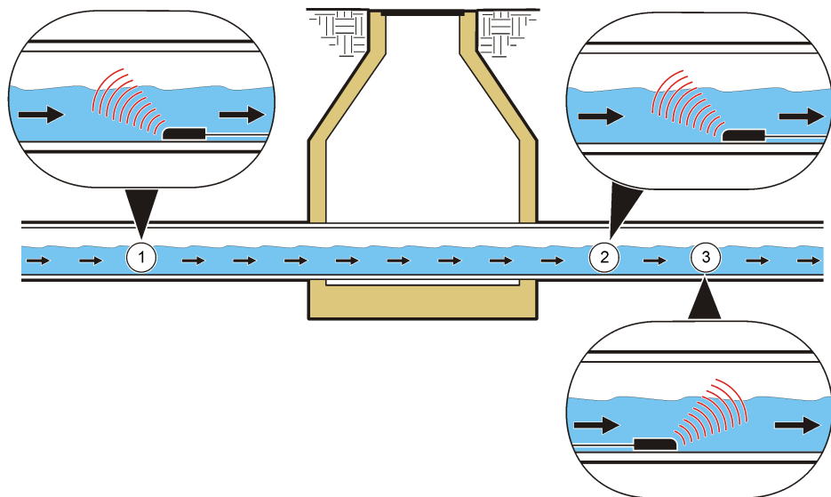
图 7 传感器位置
